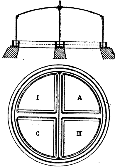
Fig. 145-146. — Valve hydraulique.
